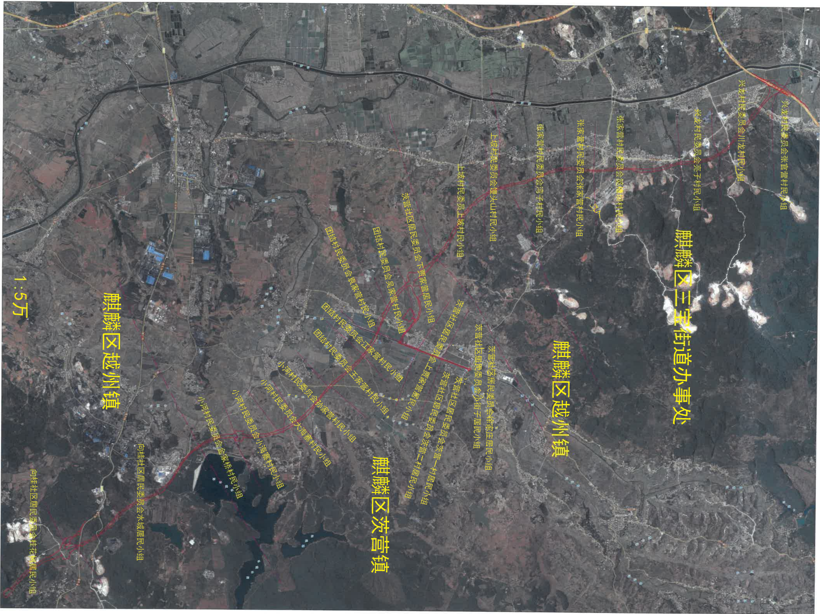
省道S11曲靖至砚山公路曲靖（麒麟区）至师宗段建设项目征地范围示意图 (起点K0+000-东山隧道K21+433)
