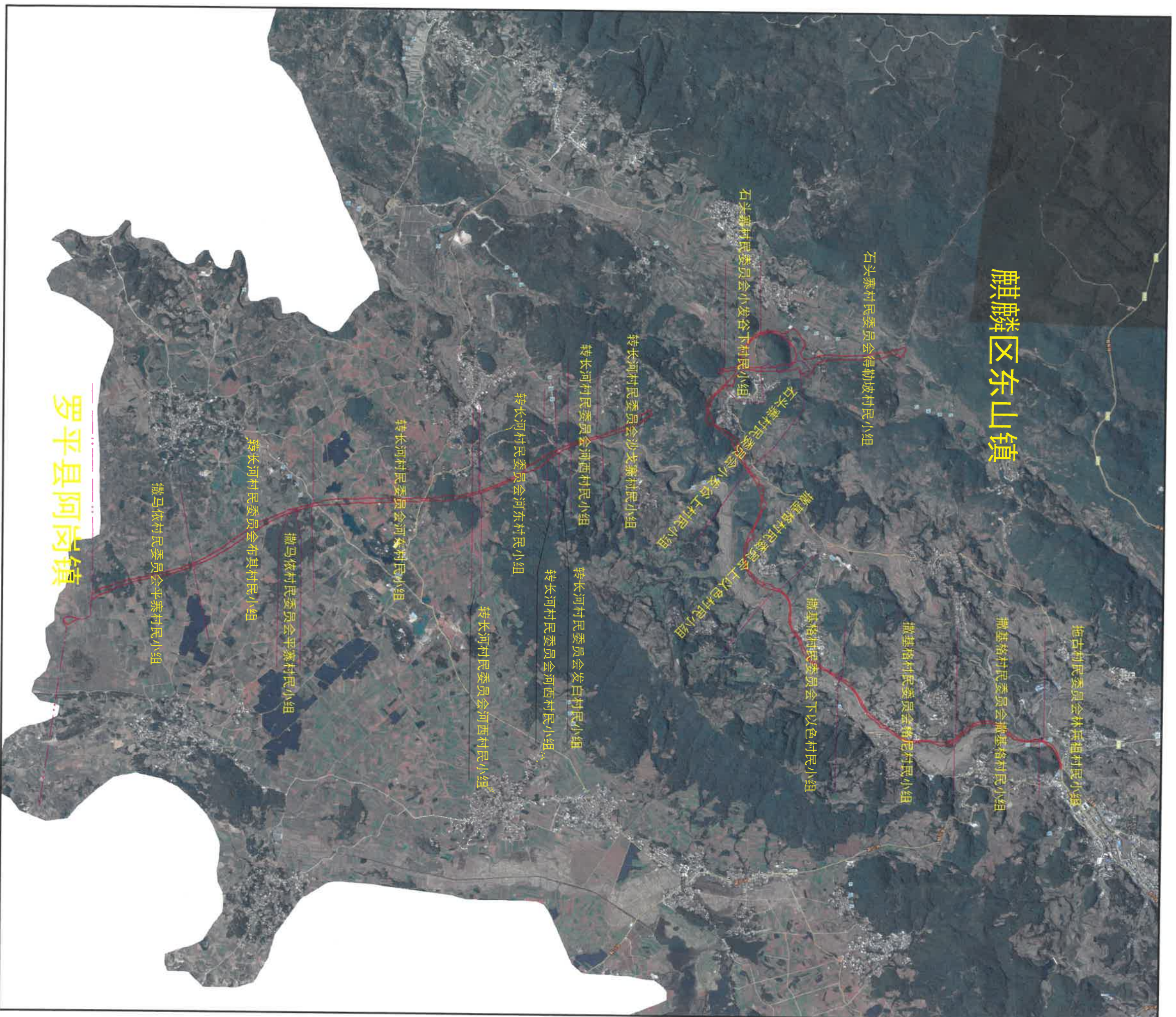
省道S11曲靖至砚山公路曲靖（麒麟区）至师宗段建设项目征地范围示意图 (东山隧道K21+433-麒麟区止点K38+668)
